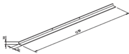
Nosný rám pre FINA (plus) F/DS, 1390 mm 1004-00568
