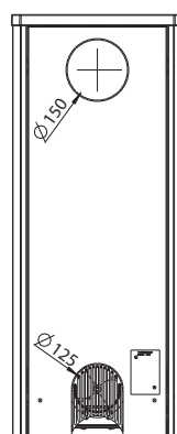
64003 dopojovacia zostava pre externý prívod vzduchu zo spodu
