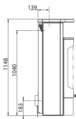
054013-xx keramický vrchný kryt, zadný vývod
