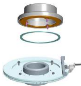
64003 dopojovacia zostava pre externý prívod vzduchu zo spodu
