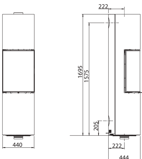
67003 zadný panel bez výre- zu pre dymovod
