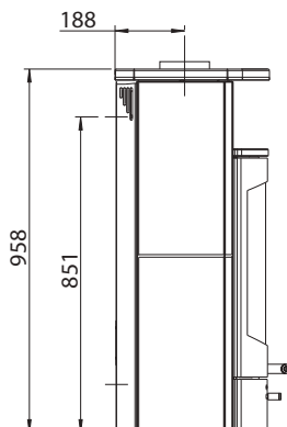
56016 prírodný kameň, zadný vývod
