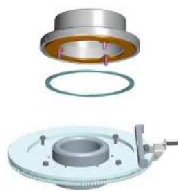
59004 dopojovacia zostava pre externý prívod vzduchu zo spodu
