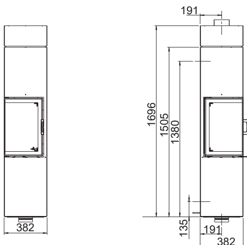
61022 otočná zostava pre ex- terný prívod vzduchu
