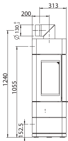
78005 HMS systém
