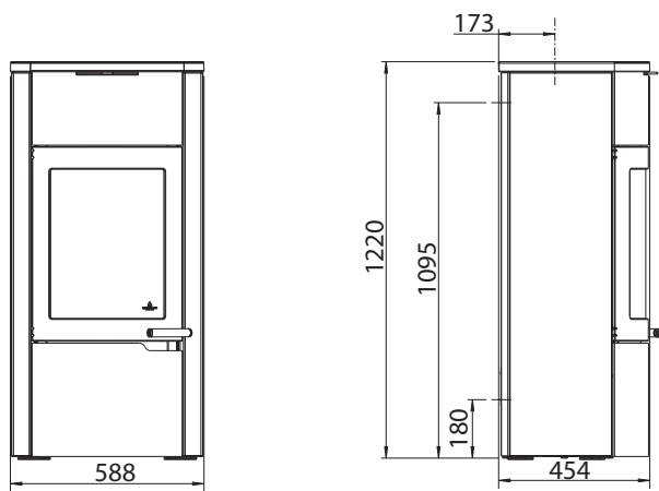
63004 mastencový vrchný kryt, horný/zadný vývod
