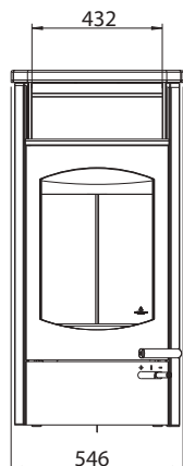
054014-xx keramický vrchný kryt, vrchný vývod
