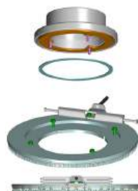
59007 otočný mechanizmus pre dymovod ø150
