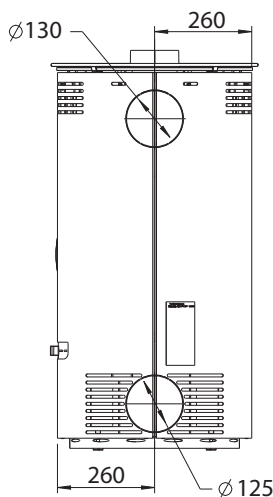
74002 adaptér pre zadné pripojenie ext. vzduchu
