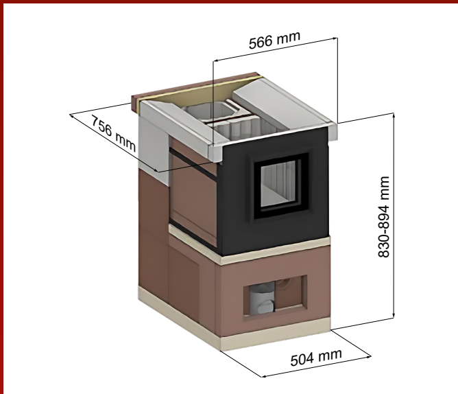
akumulačná vložka (vnútro) malého sporáka
