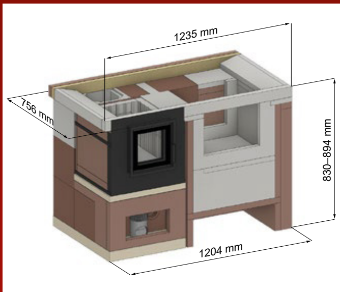
akumulačná vložka rúry (vnútro) nízka rúra
