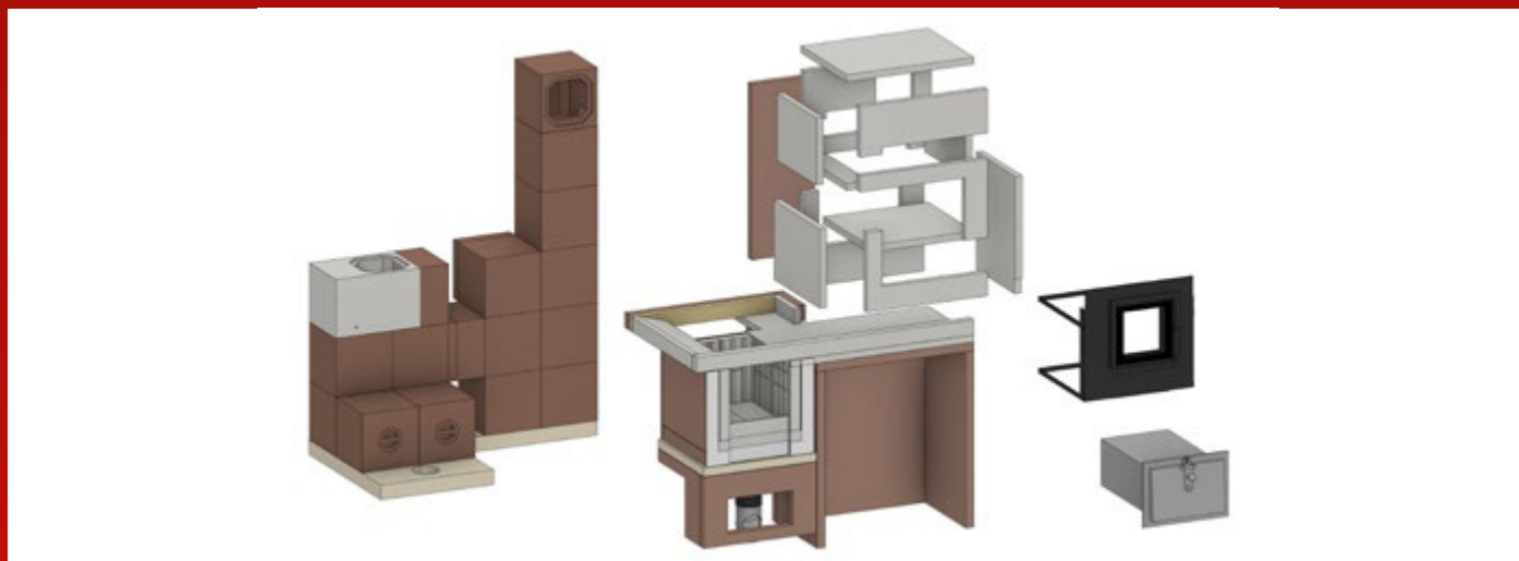
prefabrikované komponenty vysokej pece: kanálový výmenník, ohnisko s podlahovým nadstavcom a ťahmi okolo pece, čelo s dvierkami a dvojitým sklom
