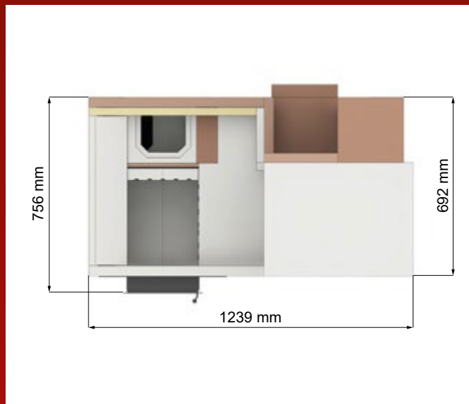
horizontálny rez vysokej vložky s rúrou
