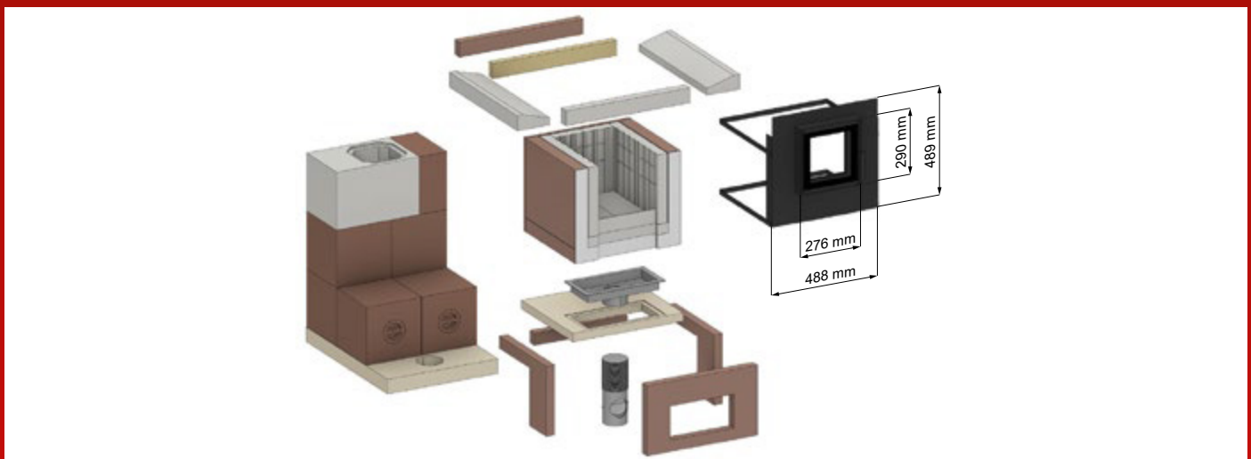
prefabrikované prvky malého sporáka: kanálový výmenník, ohnisko s podstavcom, čelo s dvierkami a dvojitým sklom
