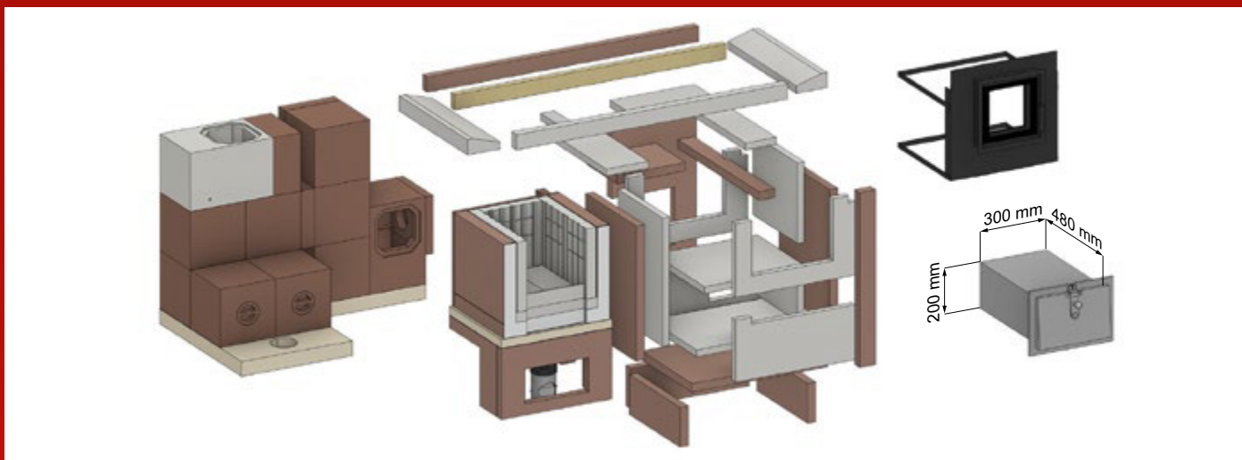
prefabrikované prvky nízkej pece: kanálový výmenník, ohnisko s podlahovým nadstavcom a ťahmi okolo pece, čelo s dvierkami a dvojitém sklom
