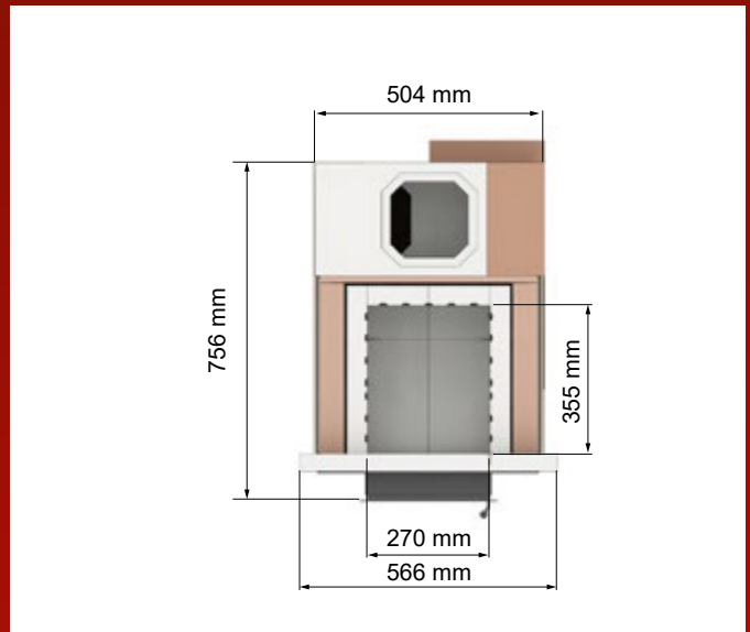
horizontálny rez vložky malého sporáka
