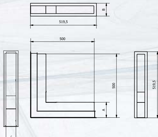
mriežka rohová s rámikom (rovnoramenná)
