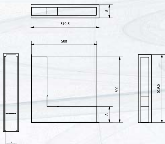
mriežka rohová bez rámika (rovnoramenná)
