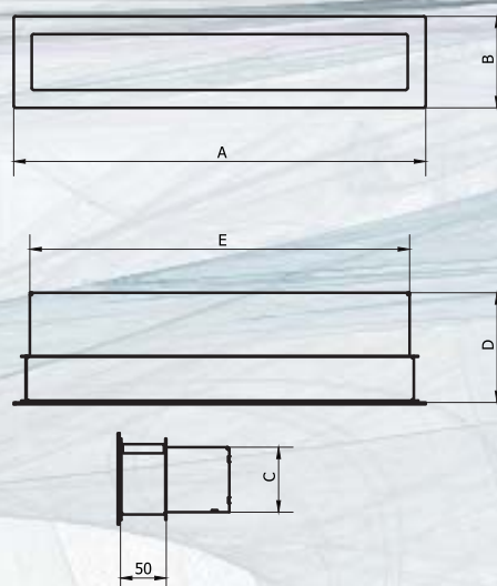
mriežka s rámikom
