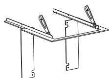
1004-01239 montážny rám s 3-stranným rámikom
