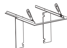
1004-01382 montážny rám s 3-stranným rámikom
