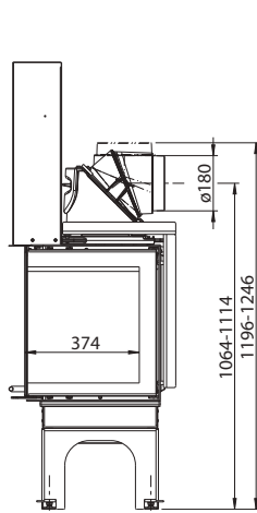
1004-01236 montážny rám s 4-stranným rámikom
