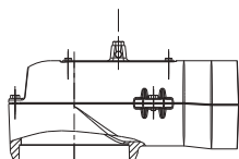
1004-00078 vyústenie, vodorovné, otočné o 360°, ø180 / ø145
