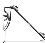
1004-01395 spojovací kus s revíz- nym otvorom - pre kombináciu s multi- funkčným hrdlom
