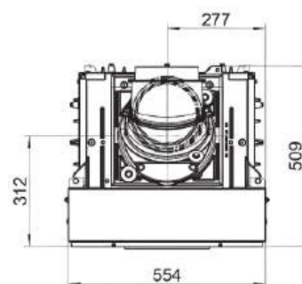
1004-01385 montážny rám s 4-stranným rámikom
