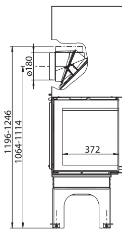
1004-01244 montážny rám s 4-stranným rámikom, ľavý
