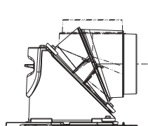
1004-01140 multifunkčné hrdlo ø180 mm
