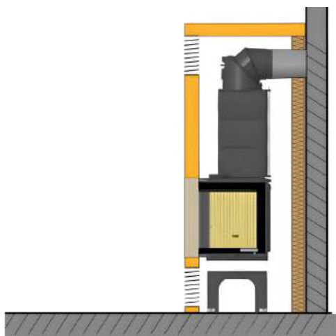
KALA s horným výmenníkom
