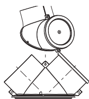
1004-00310 multifunkčné hrdlo ø180 mm dvojité s čistiacim otvorom
