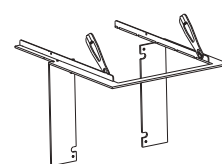
1004-01383 montážny rám s 3-stranným rámikom
