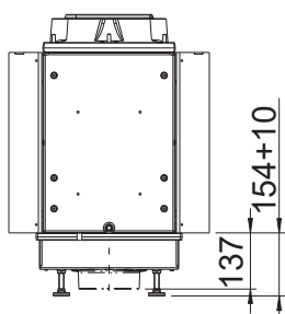
FINA na nastaviteľných nožičkách (pripojenie vonkajšieho vzduchu v spodnej časti), s nízkou montážnou výškou
