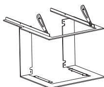
1004-01240 montážny rám s 4-stranným rámikom
