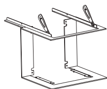
1004-01384 montážny rám s 4-stranným rámikom
