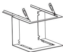
1004-01384 montážny rám s 4-stranným rámikom
