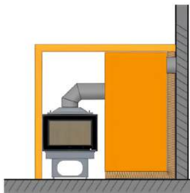
FINA plus s LWS / akumulčným ťahovým systémom
