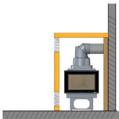
FINA s D-adaptérom pre priame pripojenie
