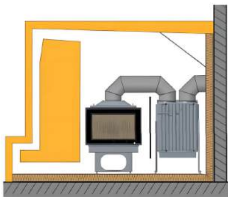
FINA plus s liatinovým výmenníkom LHK - hypokaust
