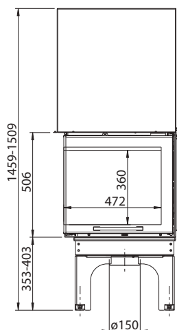
1004-01245 montážny rám s 3-stranným rámikom, ľavý
