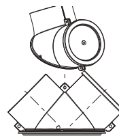
1004-00310 multifunkčné hrdlo ø180 mm dvojité s čistiacim otvorom
