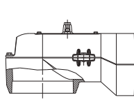
1004-00077 vyústenie, vodorovné, otočné o 360°, ø180 / ø180
