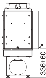
FINA na podstavci (pripojenie vonkajšieho vzduchu v spodnej časti)
