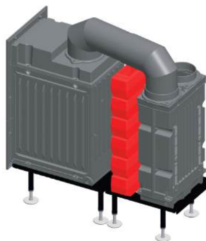
príklad použitia - pecová vložka s výmenníkom LHK so 6 LSB akumulčnými blokmi v nevyužitom priestore
