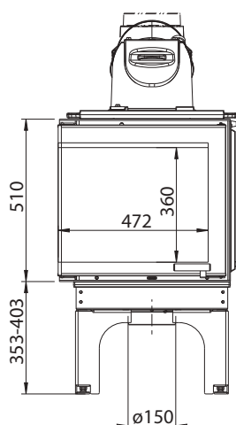
1004-01273 montážny rám s 4-stranným rámikom, ľavý
