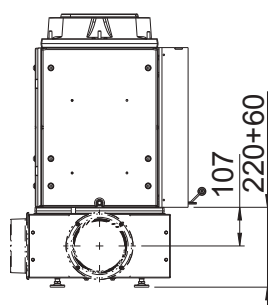
FINA so vzduchovým boxom (AIR box) (možnosť pripojenia vonkajšieho vzduchu na boku a vzadu, s nízkou montážnou výškou)
