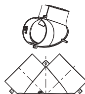
1004-00311 multifunkčné hrdlo ø180 mm dvojité s klapkou ø180/180
