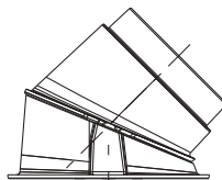
1004-01057 oceľové hrdlo pre odvod spalín, ø180 / ø200 mm
