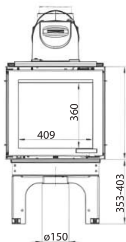
1004-01176 konvekčné opláštenie pre šírku 45 cm
