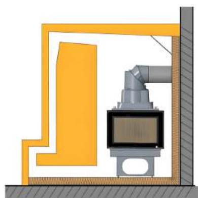
FINA ako malý hypokaust
