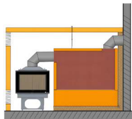
FINA plus s LWS alebo akumulčným, ťahovým systémom
