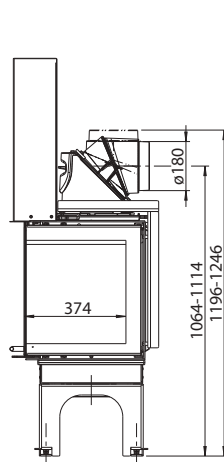
1004-01238 montážny rám s 4-stranným rámikom
