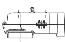
1004-01252 vyústenie, vodorovné, otočné o 360°, ø145 / ø145
