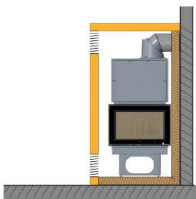
FINA s horným výmenníkom tepla
