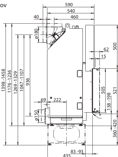
1004-01104 LWS Set 3, 7 elementov
