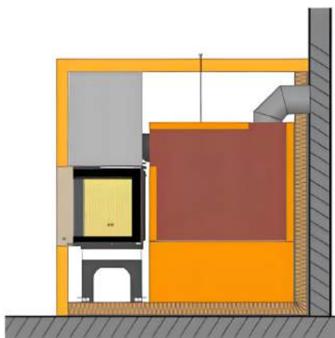
KALA s LWS alebo keramickým ťahovým systémom
