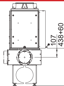
FINA s airboxom + podstavec (pripojka vonkajšieho vzduchu na boku, možnosť zadnej/prednej časti), pre väčšie inštalačné rozmery
