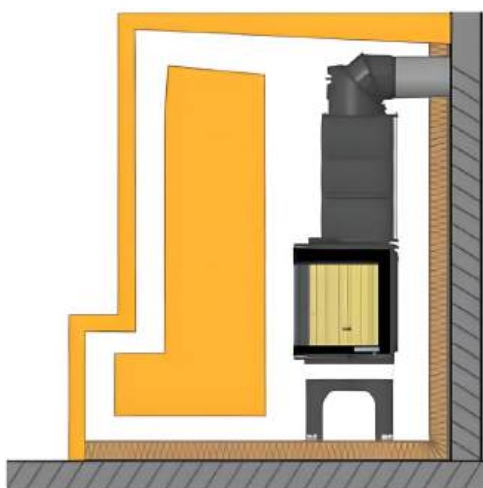
KALA ako hypokaust s horným výmenníkom
