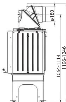
1004-01177 konvekčné opláštenie pre šírku 55 cm
