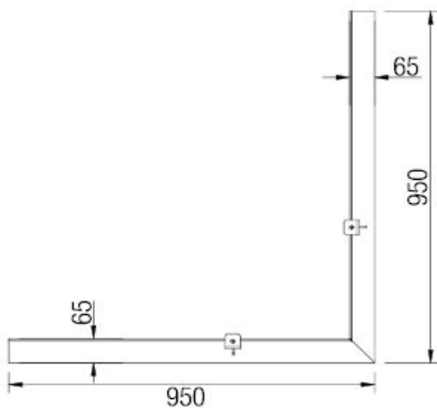
354009 / oceľ, d95 cm, š6 cm
