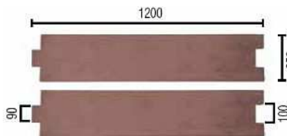
350147 / šamot, d120 cm, š6 cm, 2 diely
