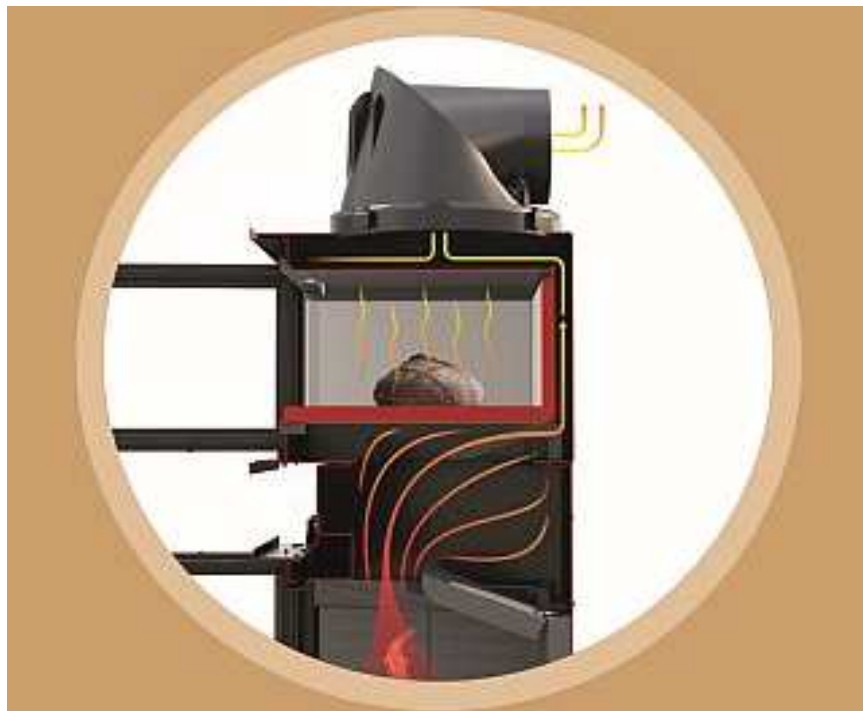
technológia vedenia spalín
