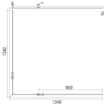
358060 / oceľ, d134 cm, š5 cm
