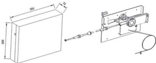
363010 / Regulácia horenia InsertControl
